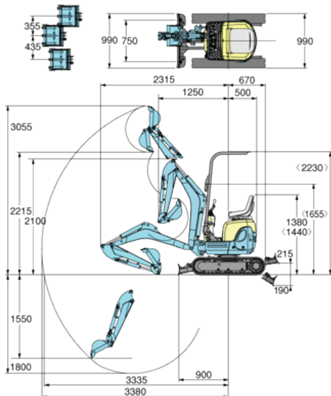
■作業範囲図 単位：mm
