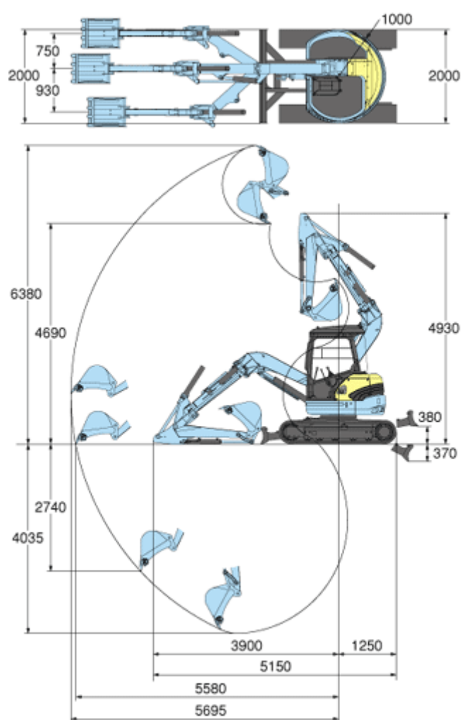
■作業範囲図 単位:mm
